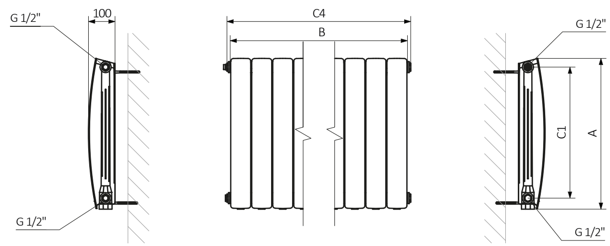
A - Hauteur B - Largeur C1, C4 - Espacement des connexions
